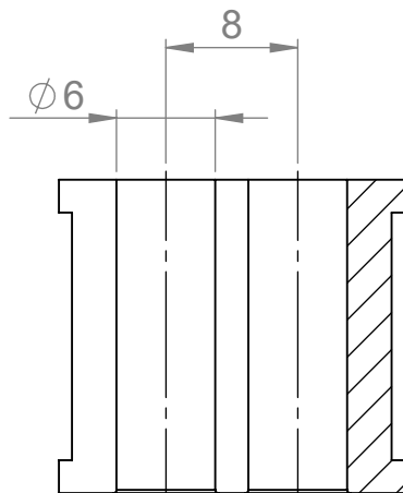
SCHNITT A-A
