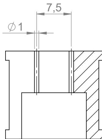
SCHNITT A-A
