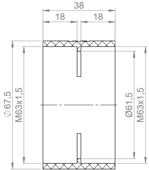
SCHNITT A-A
